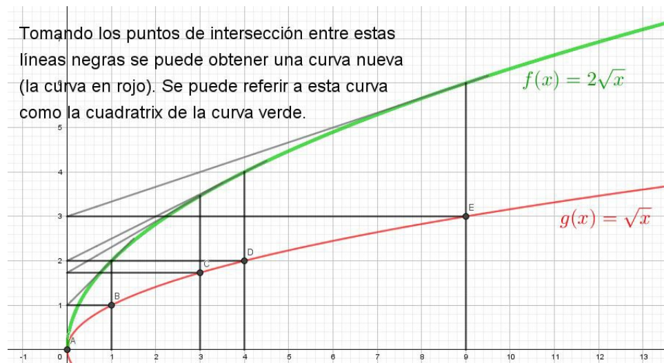
Figura 3. Construcción de la quadratrix (en rojo) a partir de la curva original (en verde)
