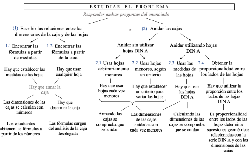
Figura 2. Esquemas identificados en la situación de estudio.
