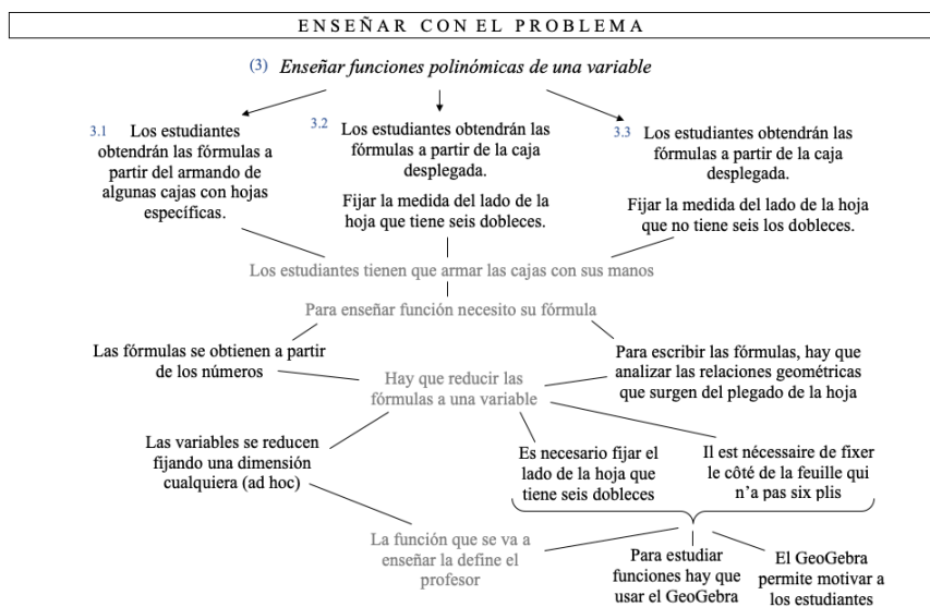
Figura 3. Esquemas identificados en la situación de enseñanza sobre las funciones polinómicas.
