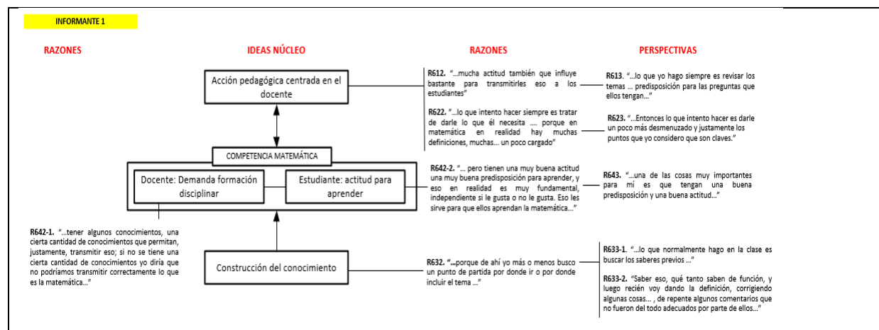
Figura 2. Mapa cognitivo, que describe el sistema de creencias del informante 1, en relación con la categoría Competencia Matemática.
