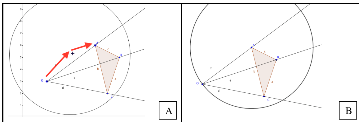
Figura 6 - a) Arreste da circunferência criada pelo compasso, b) fixação da circunferência translada para o ponto A.
